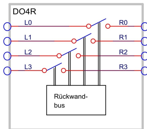
Blockschaltbild der DO4-R
