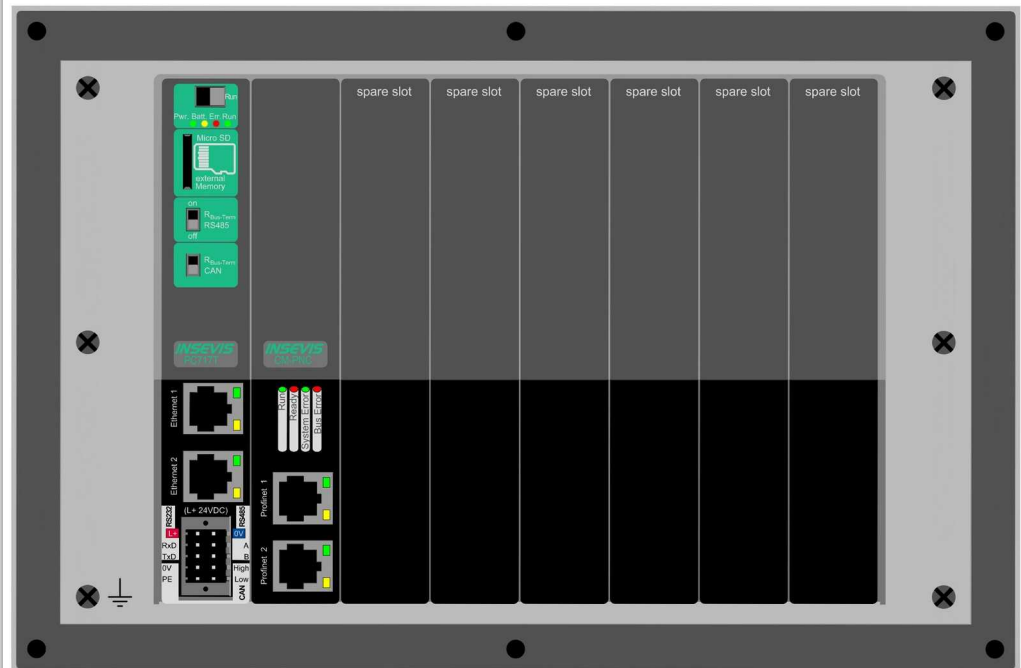
Bild oben: Ansichten der Anschlusseiten PC717T-PNC von hinten
