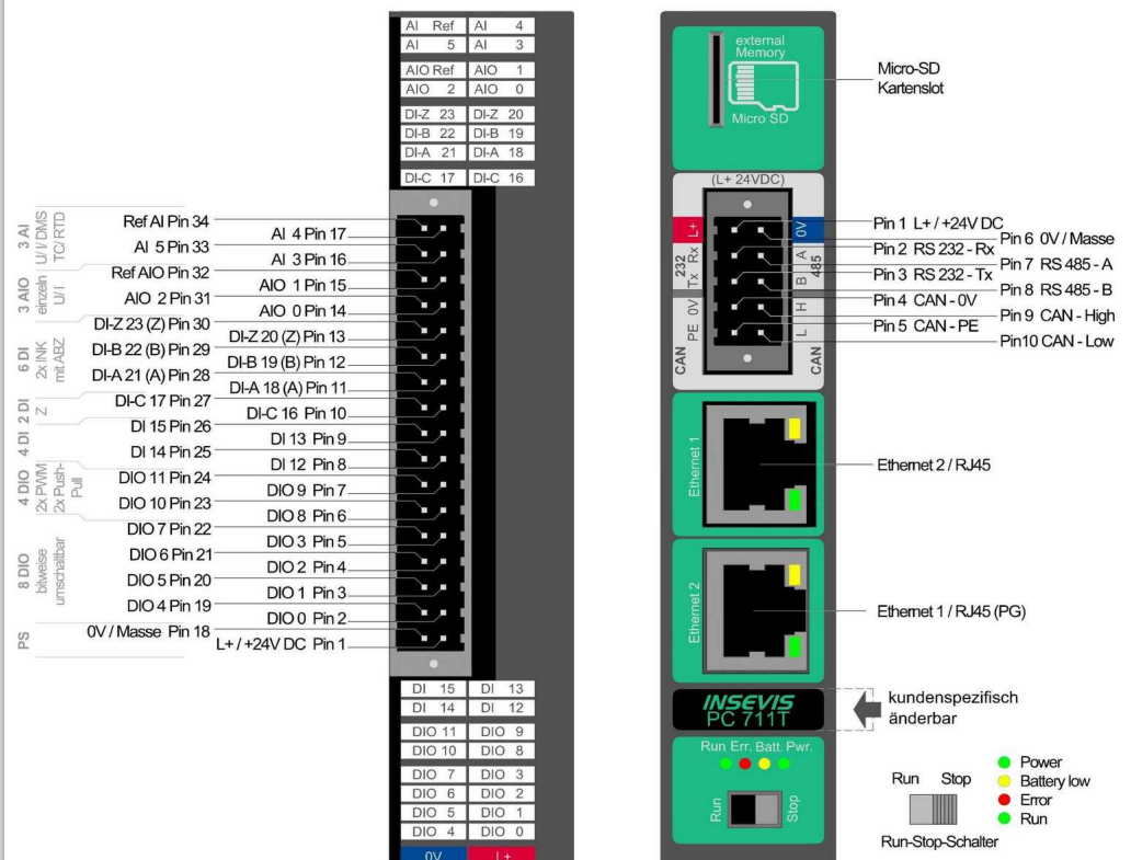
Bild oben: Beschriftung der CPU-Anschlüsse aller Panel-SPS PC711T
