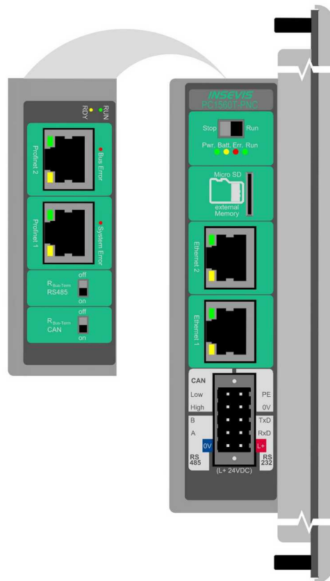
Bild oben: Ansichten der Anschlusseiten PC1560T-PNC (an der rechten Seite und oben)
