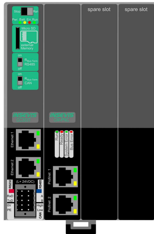
Bild oben: Ansichten der Anschlusseiten CC303T-PNC
