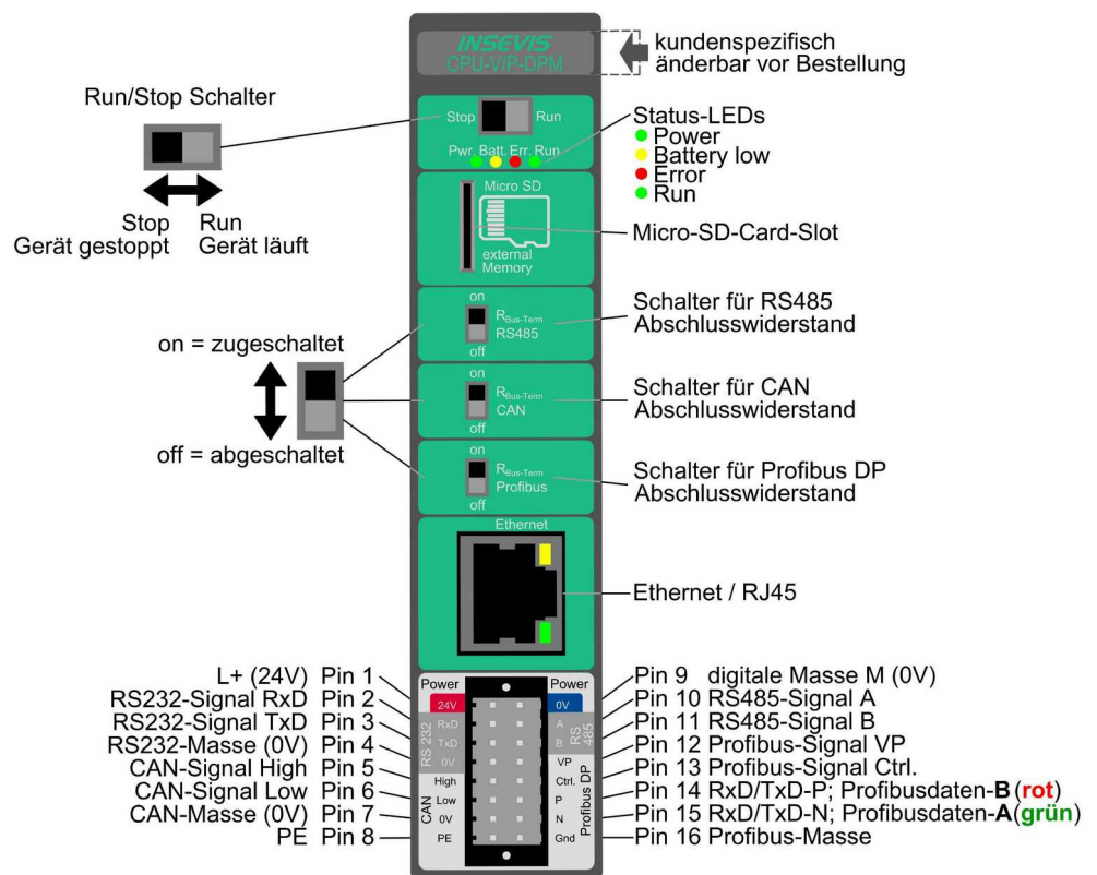
Bild oben: Beschriftung der CPU-Anschlüsse des Kompakt-SPS-Grundgerätes mit der CPU Typ V und mit Profibus DP-Master
